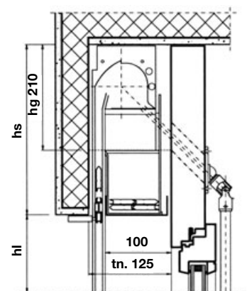
Sezione verticale
