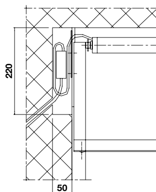
Dettaglio visto interno con comando a motore
