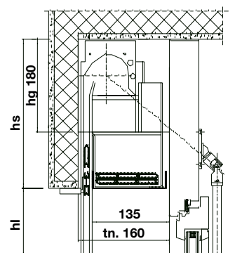
Sezione verticale
