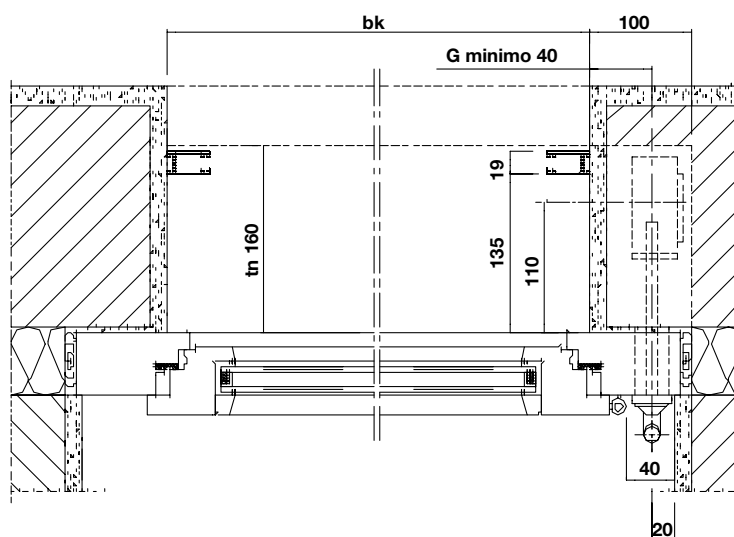
Sezione orizzontale
